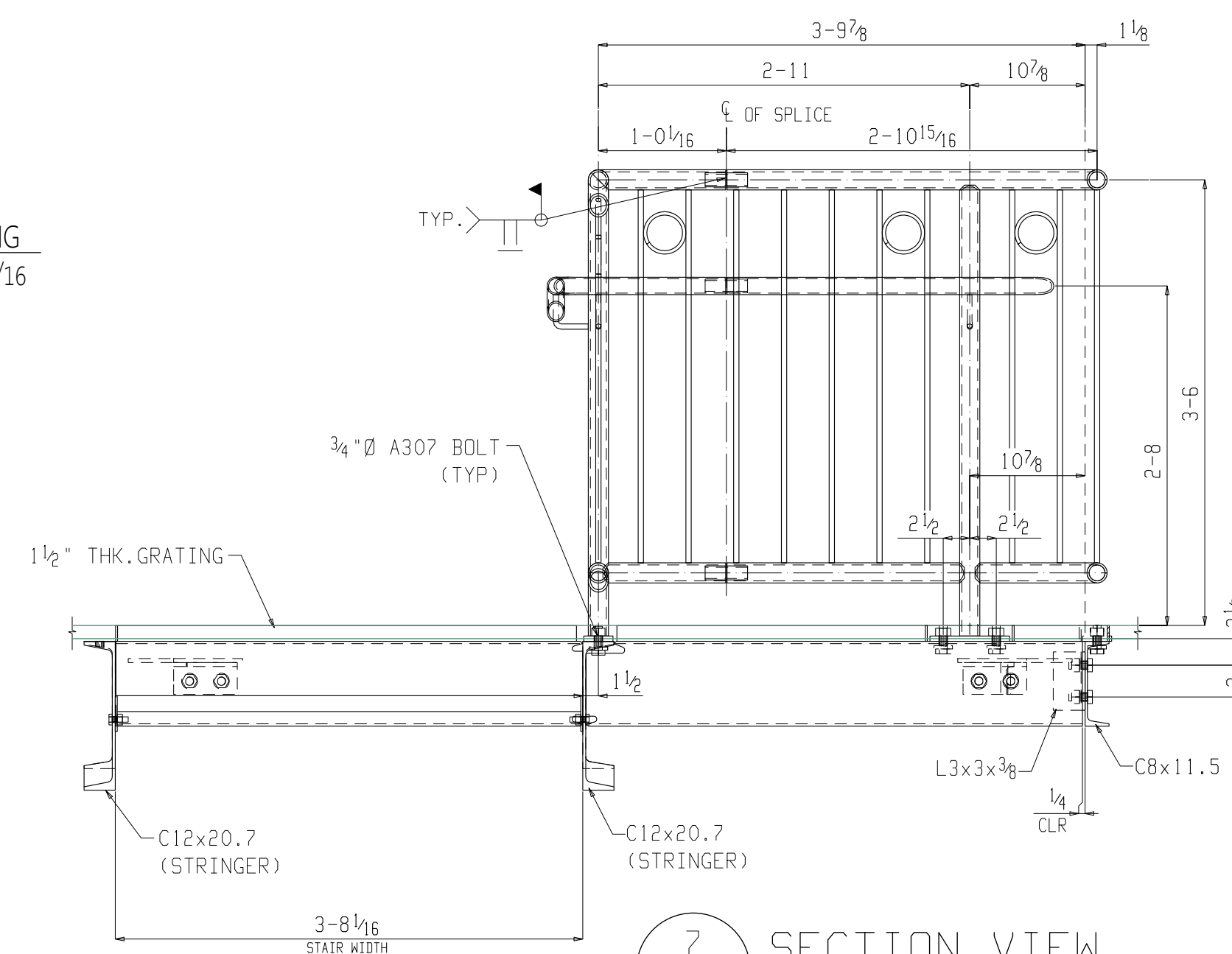
7 E3 SECTION VIEW
