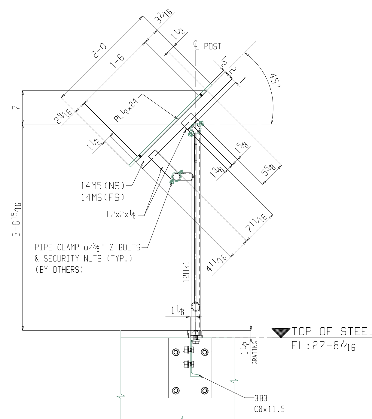
11 E3 SECTION VIEW
