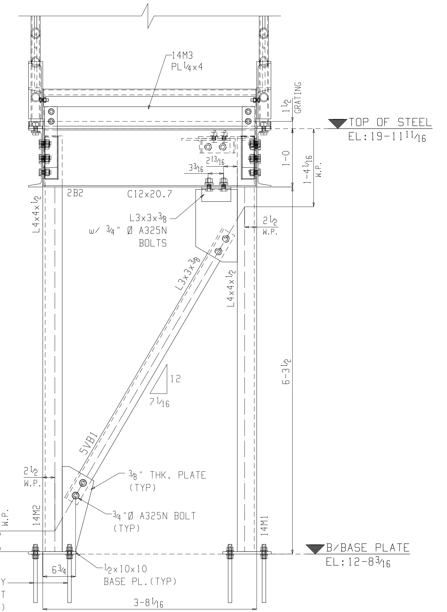
8 E3 SECTION VIEW
