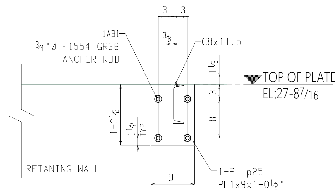
5 E3 SECTION VIEW (REF.DRW. E/A58)
