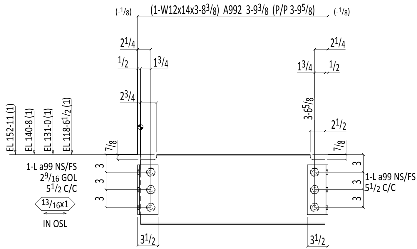
4 BEAMS 215B2
