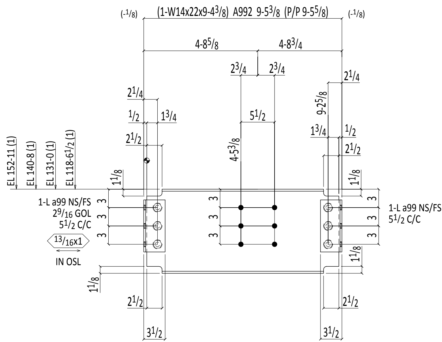
4 BEAMS 215B4
