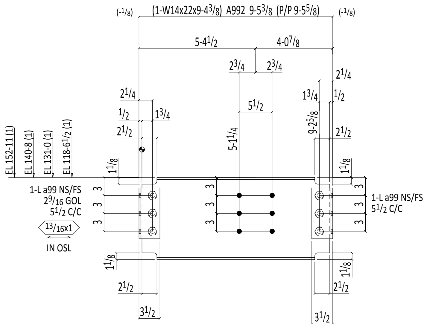
4 BEAMS 215B5
